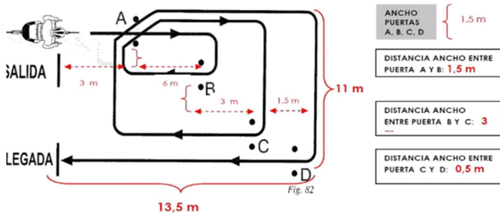
Il·lustració 1: Esquema Remolí excèntric
